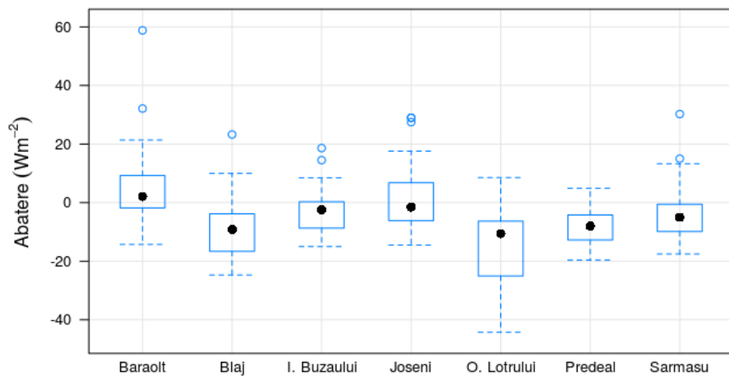
Diagrama de tip boxplot a abaterilor lunare dintre radiația solară globală măsurată și SIS-SARAH (2012-2014).
