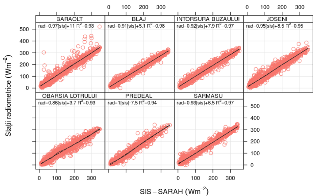
Graficul de corelație de tip puncte și coeficienții de determinare R^2 dintre datele zilnice de radiație globală măsurate și SIS-SARAH (2012-2014).
