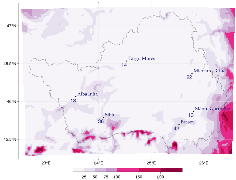
Harta densității energiei eoliene ( Wm^{-2} ) la 10 m înălțime deasupra solului
