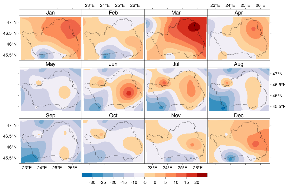
Regiunea 7 Centru: abateri ( Wm^{-2} ) medii lunare multianuale (2012-2014) dintre radiația solară globală măsurată și SIS-SARAH.
