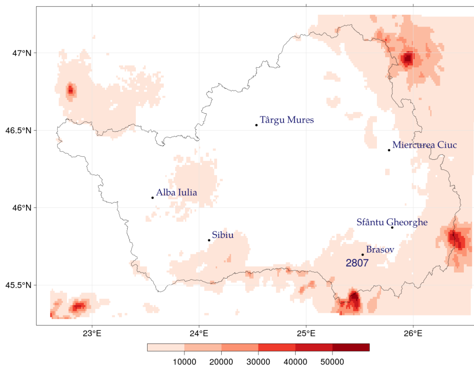
Regiunea 7 Centru: estimarea producției anuale de energie (kWh) pentru o turbină cu trei pale, cu o putere 10.4 kW@11 m/s, instalată la 24.4 m înălțime deasupra solului.
