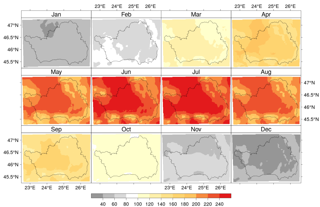
Regiunea 7 Centru: radiație solară globală (Wm -2 ) extrasă din produsul SIS-SARAH, medii lunare multianuale (1983-2012).
