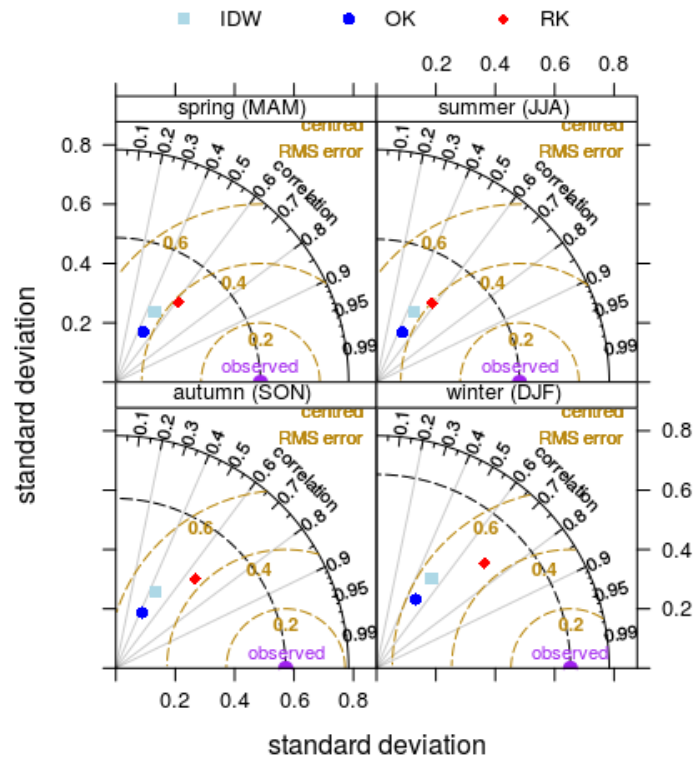
Diagrame sezoniere de tip Taylor: seturile de date de vânt estimate prin procedura de validare încrucișată utilizând metodele de interpolare IDW, OK și RK vs. date observate.
