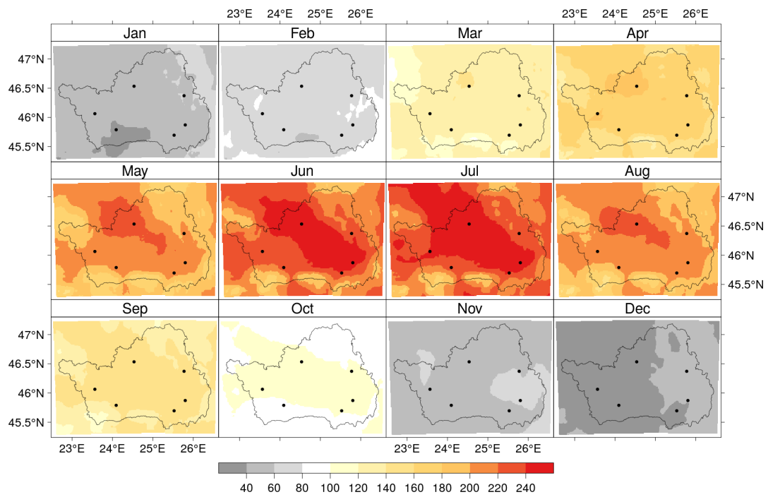
Regiunea 7 Centru: radiație solară globală (Wm -2 ) medii lunare multianuale (1983-2012).
